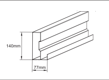
ビーム
